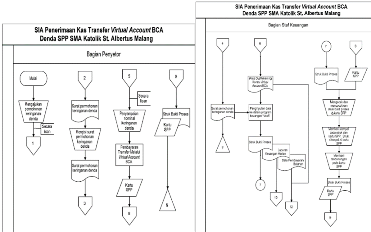
Gambar 2. Usulan Bagan Alir SIA Penerimaan Kas Transfer Virtual Account BCA Keringanan Denda SPP
