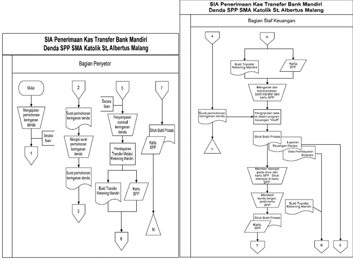
Gambar 3. Usulan Bagan Alir SIA Penerimaan Kas Transfer Bank Mandiri Keringanan Denda SPP
